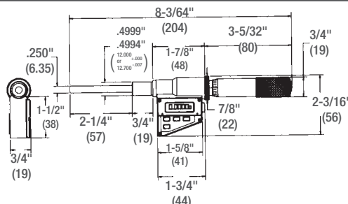
0-2" (0-50mm) dimensions
